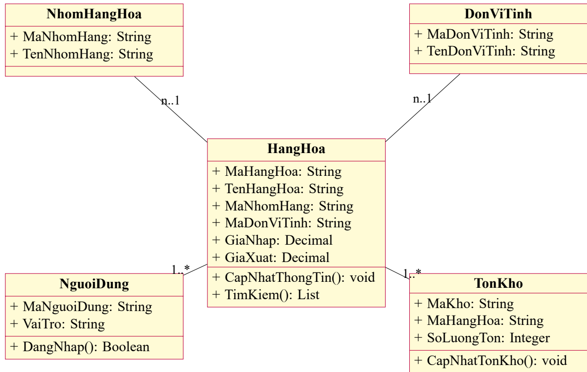
Hình 6.4: Biểu đồ lớp trong ca sử dụng UC15 – Thêm hàng hóa
