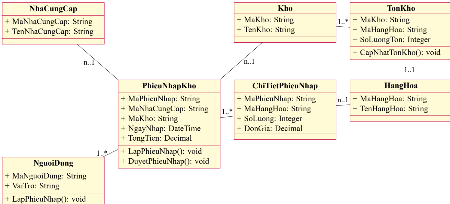
Hình 6.5: Biểu đồ lớp trong ca sử dụng UC22 – Lập phiếu nhập kho
