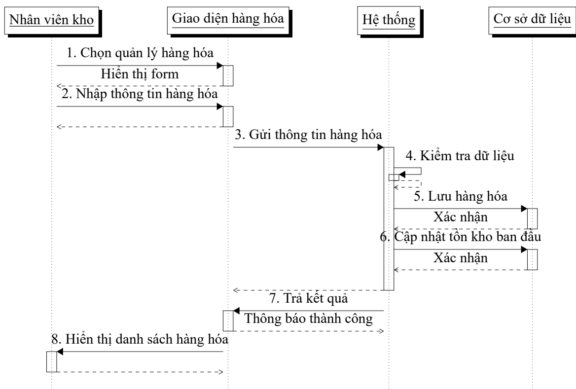
Hình 5.1: Sequence diagram UC15 – Thêm hàng hóa
