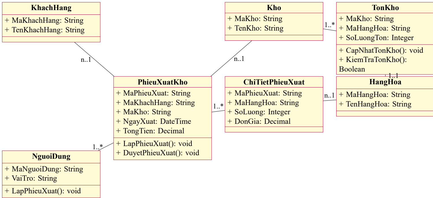
Hình 6.6: Biểu đồ lớp trong ca sử dụng UC24 – Lập phiếu xuất kho
